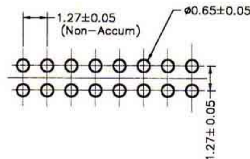
P.C.B. LAYOUT
